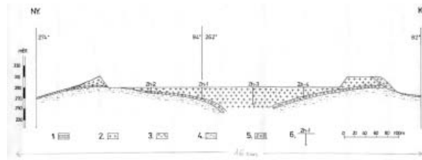
4. ábra. A zalahalápi bazalt bánya nyugat-kelet irányú földtani szelvénye. 1 - bazalttörmelék, humuszos termőtalaj, 2 - felső-pliocén bazalt, 3 - felső-pliocén piroklasztikum, 4 - felső-pannoniai agyagos homok, 5 - meddőhányó, 6 - kutatófúrás.
